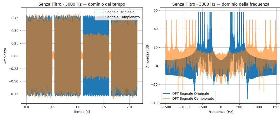
Figura 6: Confronto tra il segnale originale (blu) e il segnale con rumore (arancione) campionato a 3000 Hz senza filtro. A sinistra, il segnale nel dominio del tempo; a destra, l'analisi nel dominio delle frequenze mostra chiaramente gli effetti del rumore e l'aliasing nel segnale campionato.
