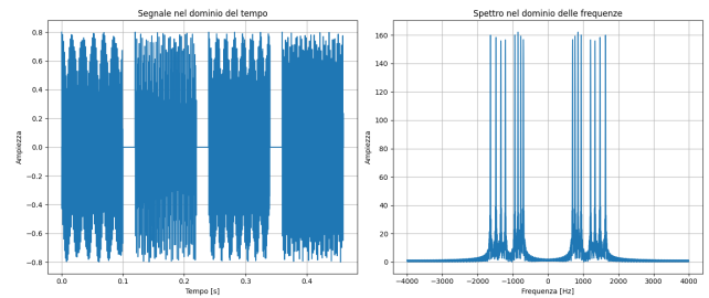
Figura 4: Segnale nel dominio del tempo e frequenza per una durata di 0.1 s (sequenza "2 4 C #").
